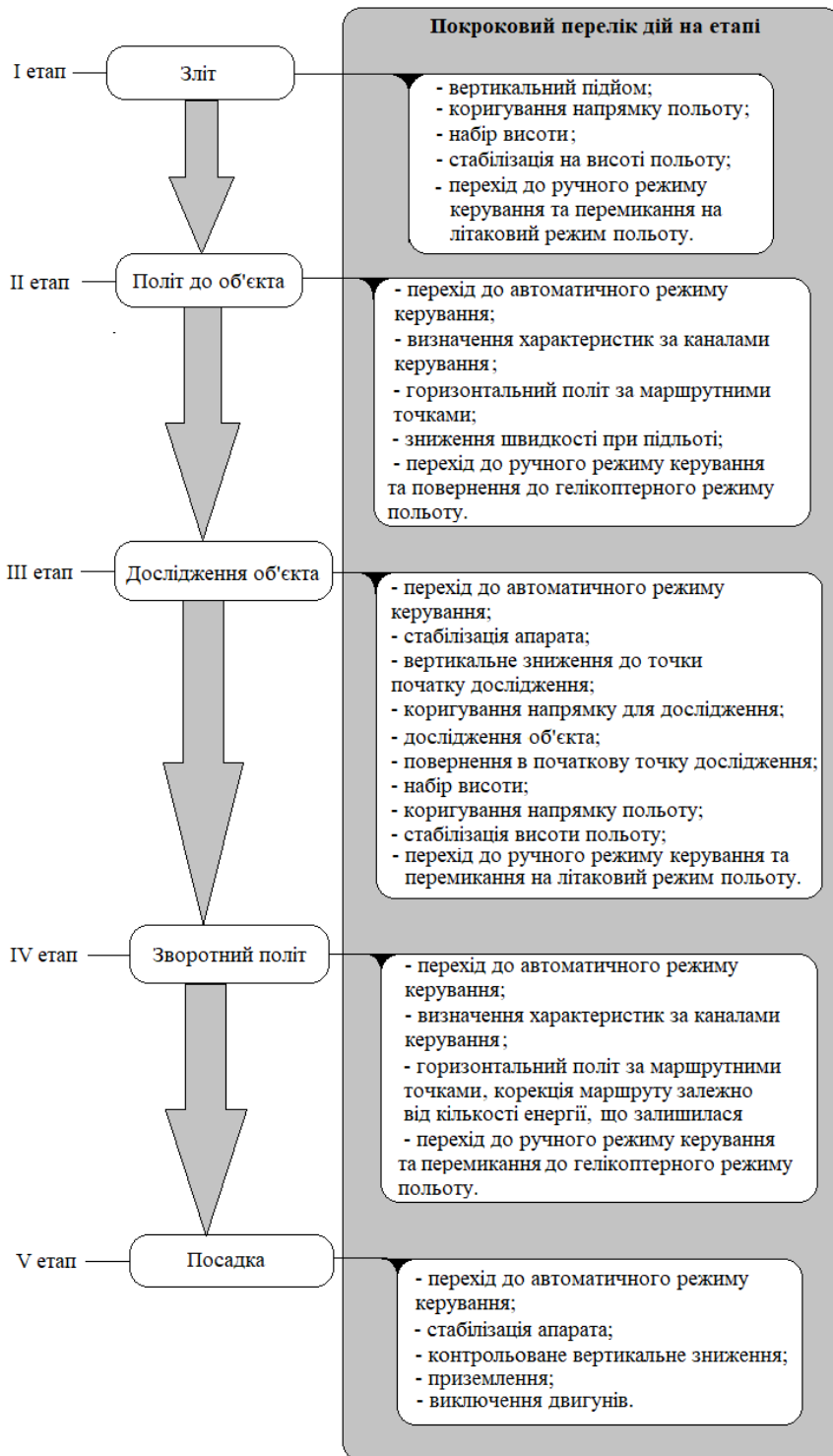
Рис. 2. Блок-схема методу комбінованого керування рухом гібридного безпілотного літального апарата.
